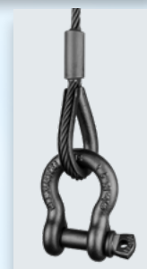
Exemple d'application. Manilles voir p.27
